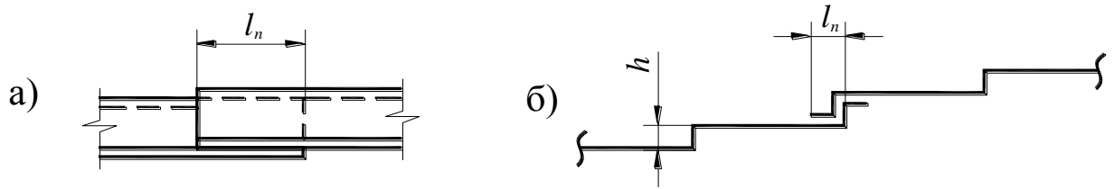
Рисунок 5 – Кінцеві поперечні стики: а – для виробів будь-якого типу; б – за конструктивним вирішенням ( l_n – величина напуску, h_r – висота гребеня, l – довжина приступки, або крок гребенів)
