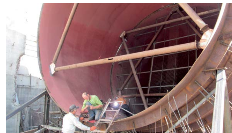
Изготовление и монтаж водоводов D=7,5 м – 2 800 т
