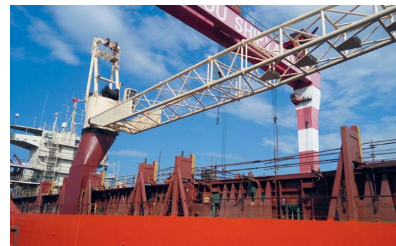
□ Ремонт т/х Ocean Lord, Китай
