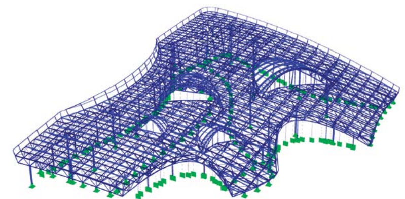
□ Крыша водного центра в Куршевеле
