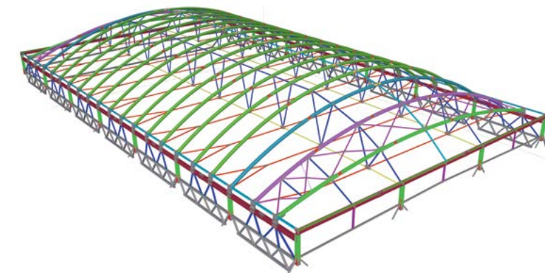
□ Проект ТРЦ RETROVILLE, г. Киев, Украина
