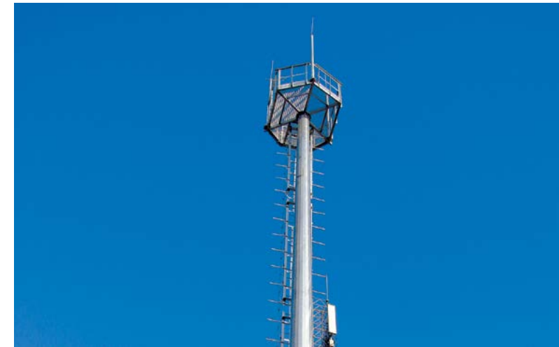
□ Мачты связи на основе МГС от 25 до 40 м, МТС, Lifecell, Украина
